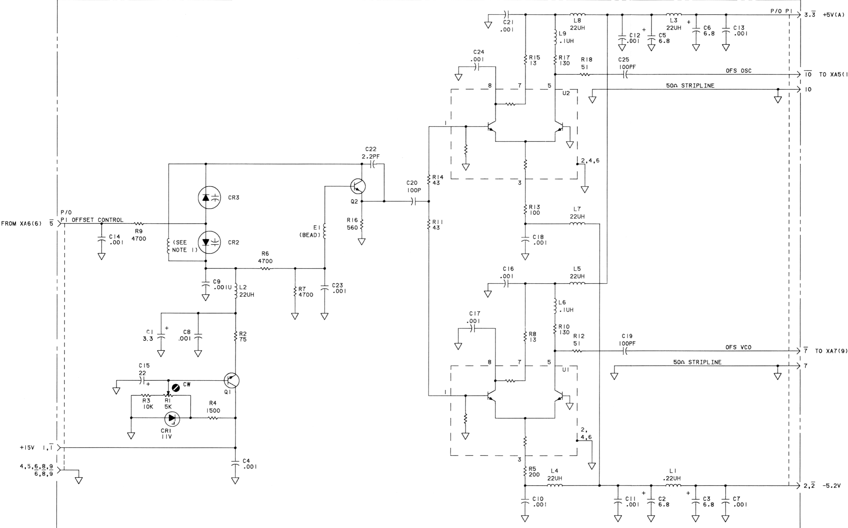
Figure 8-27. A4 Offset VCO Assembly
